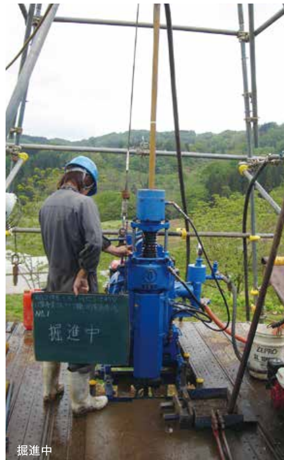
仮設足場状況
