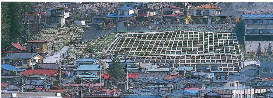
急傾斜地災害復旧工事(下諏訪東町)
