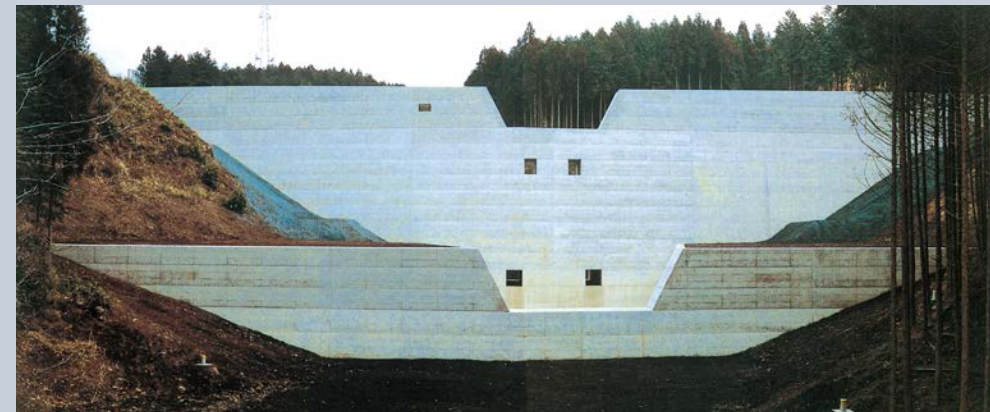
国土交通省・富士山久遠寺第2砂防ダム・富士宮市
